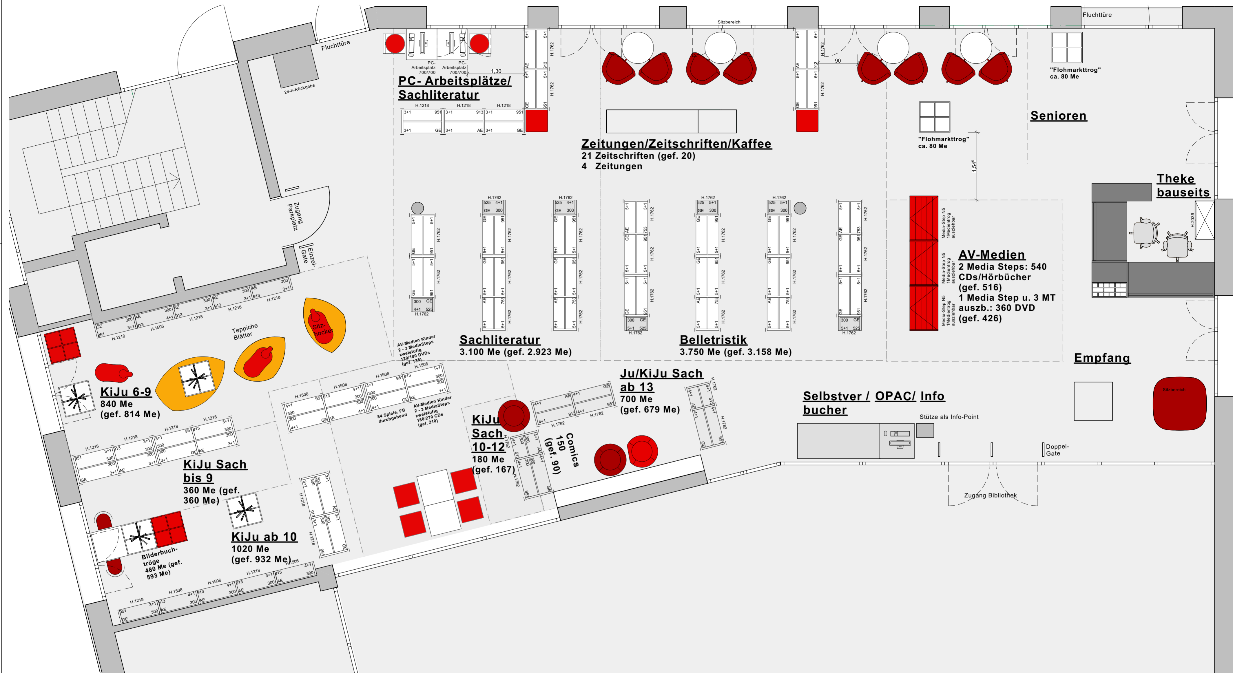
Grundriss
