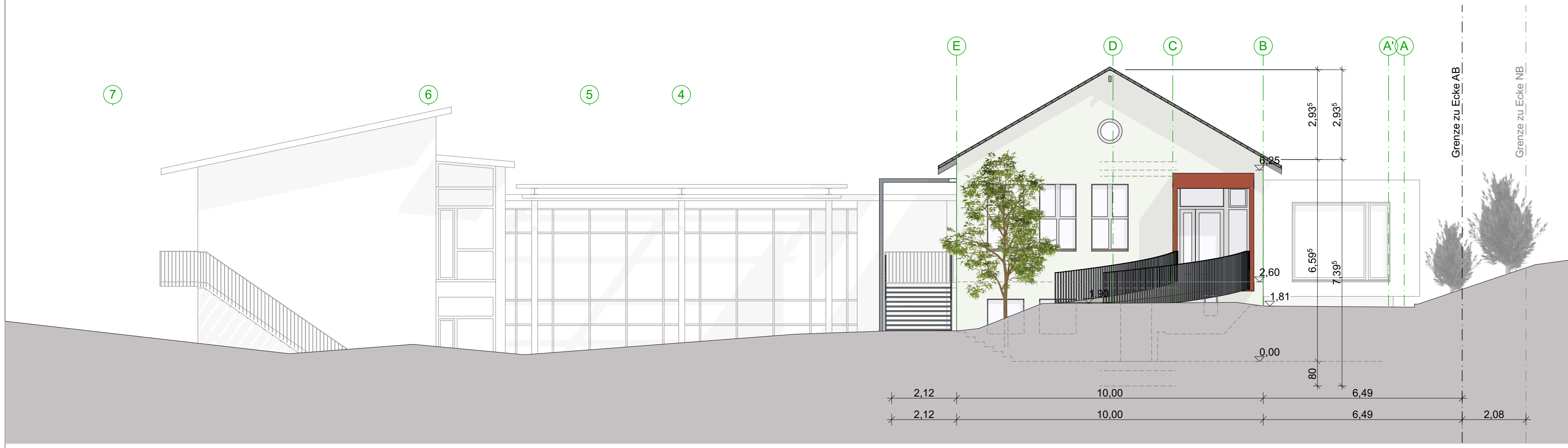
Ansicht Ost
