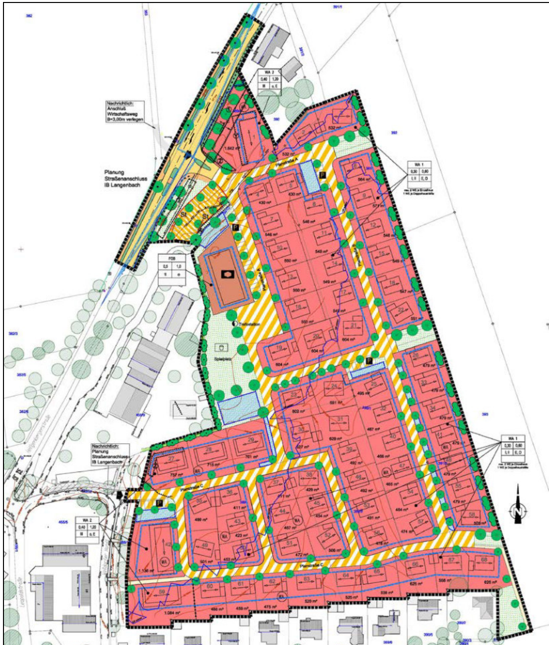
Rechtsplan des Bebauungsplanes (Ausschnitt ohne Maßstab)
